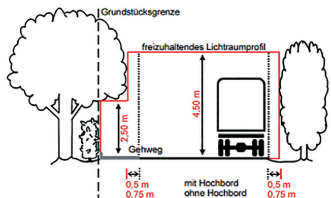
Abbildung: Lichtraumprofil für Straßen und Gehwege
