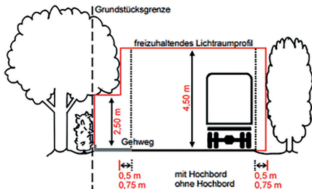
Abbildung: Lichtraumprofil für Straßen und Gehwege
